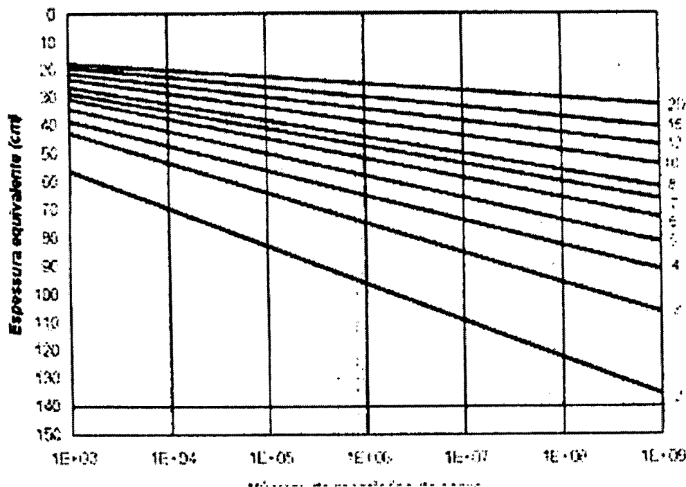
Ábaco de Dimensionamento de Pavimento Flexível Método DNER-1966/79
